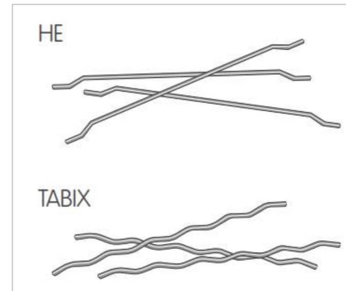
Hình dạng sợi thép Móc hai đầu và Gợn sóng
