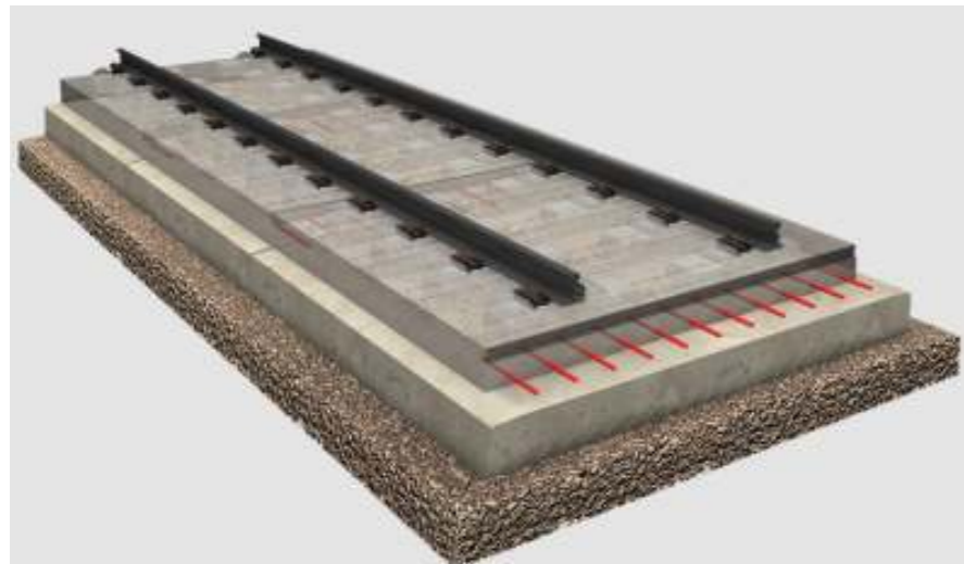
Kết cấu sàn bê tông đỡ ray đường sắt
